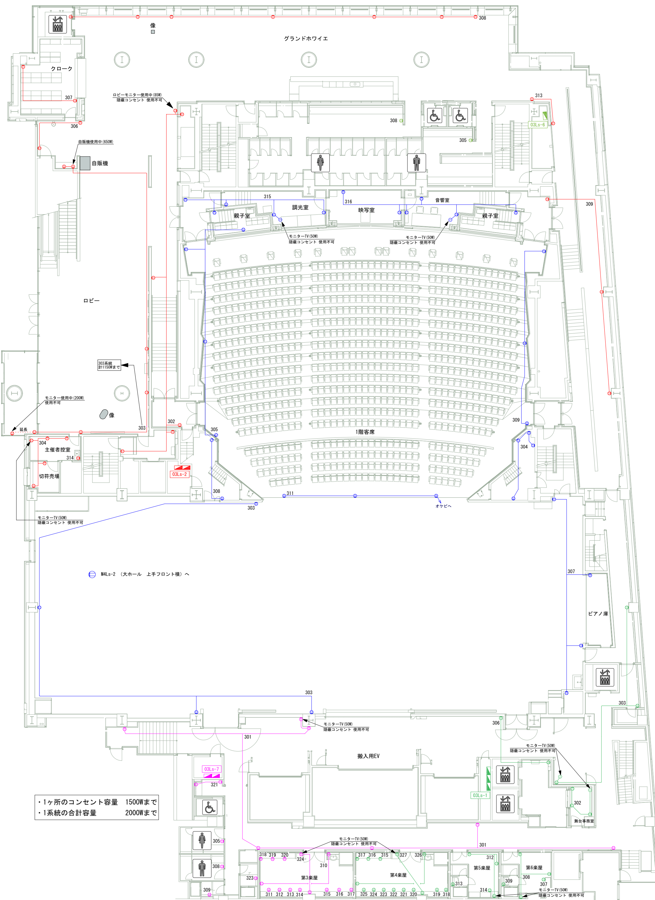
サンポートホール高松 大ホール電気系統図 (3F) A3:1/200
